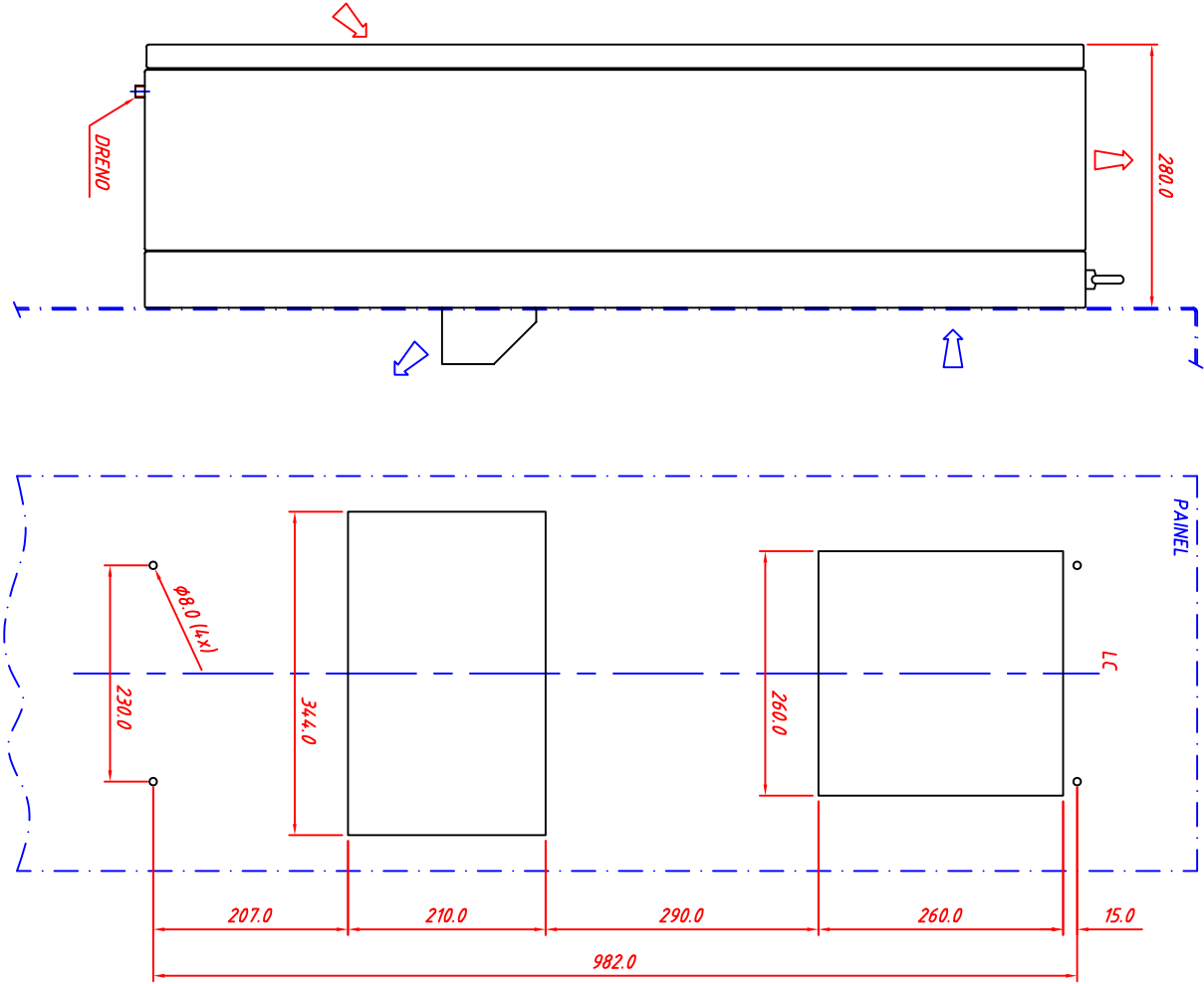
MONTAGEM EXTERNA
