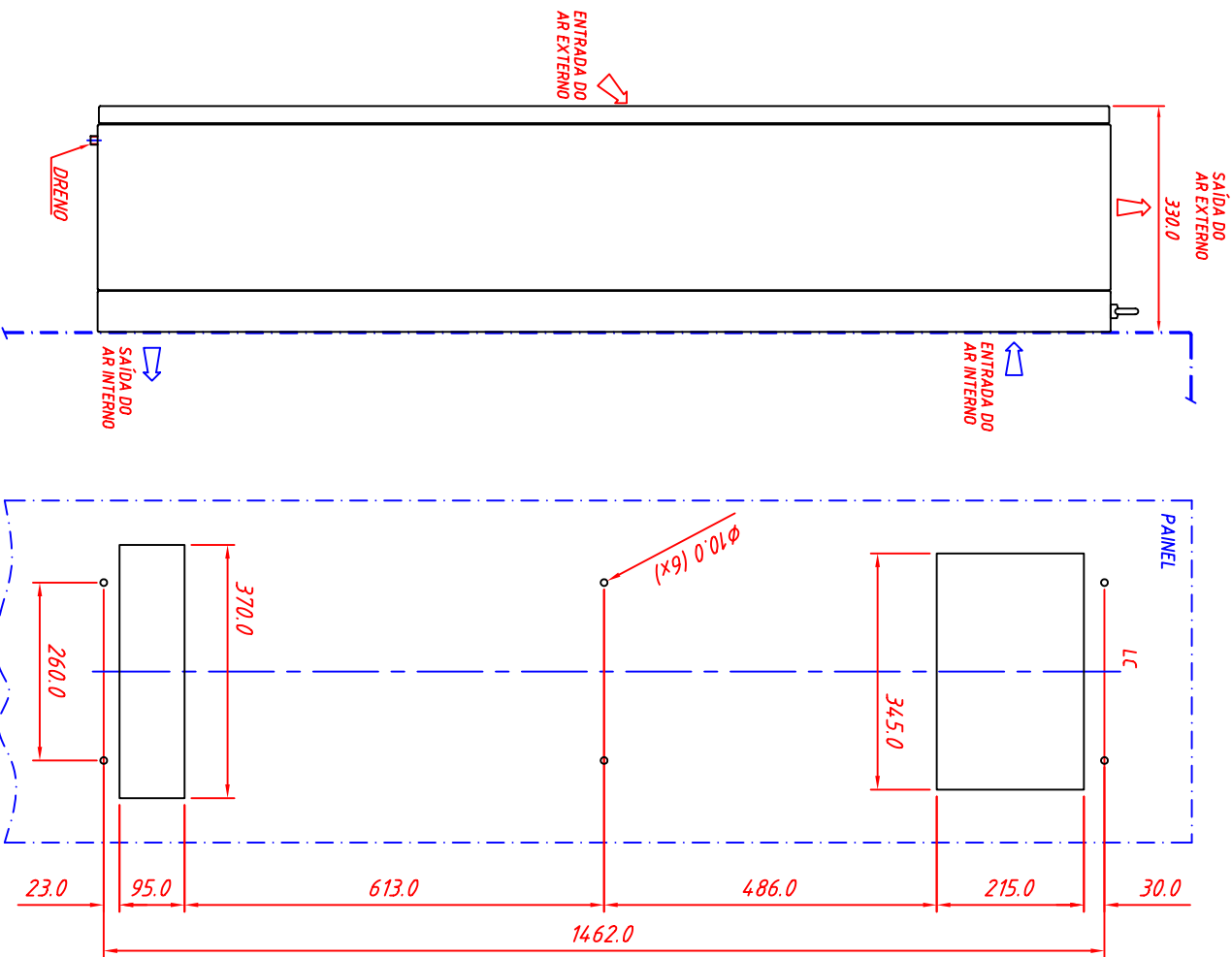
RECORTES E FURAÇÕES P/ INSTALAÇÃO (MONTAGEM EXTERNA)
