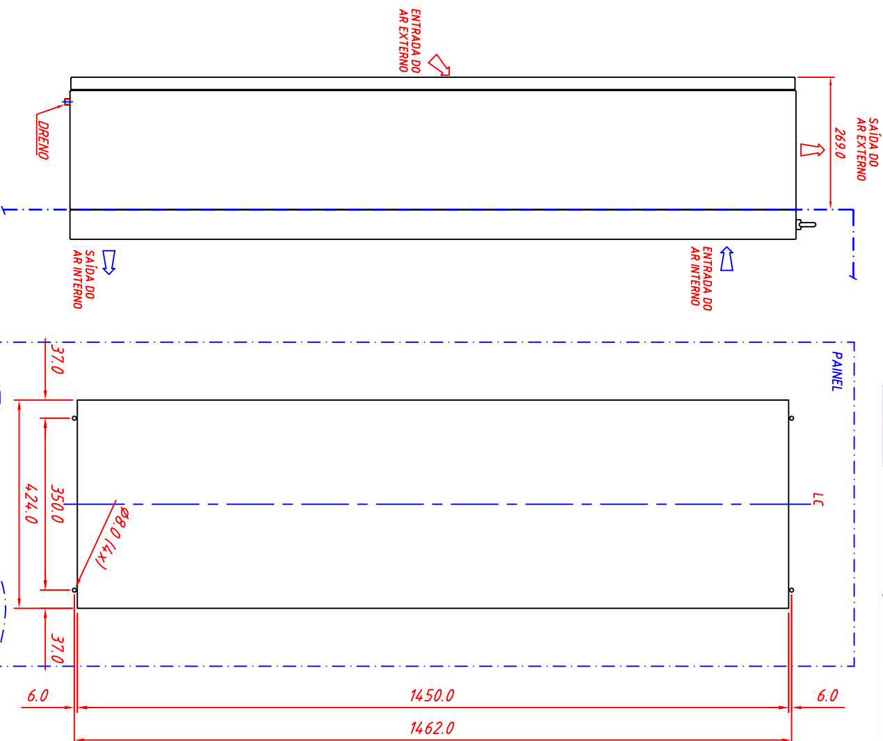
RECORTE E FURAÇÕES P/ INSTALAÇÃO (MONTAGEM SEMI-EMBUTIDA)
